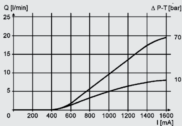
Q 08 spool
