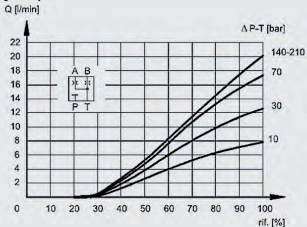
Q 08 spool
