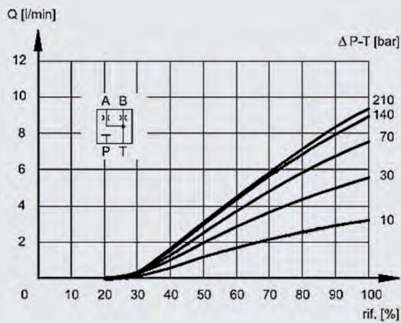
Q 04 spool
