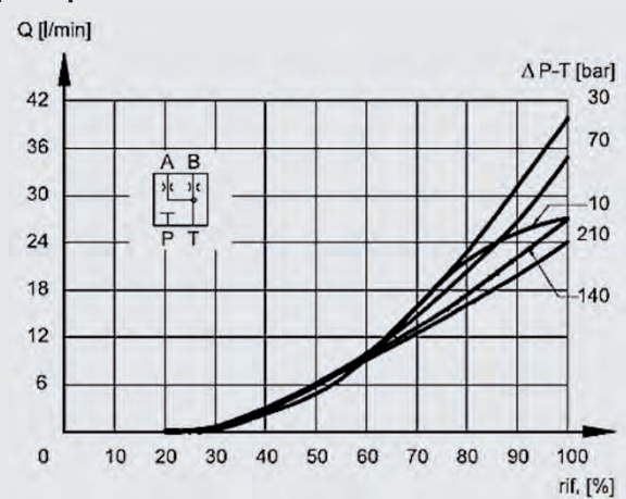
Q 26 spool
