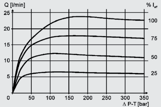
Q 16 spool
