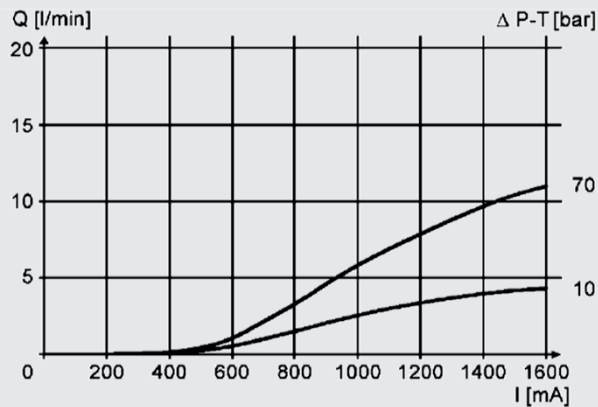
Q 04 spool
