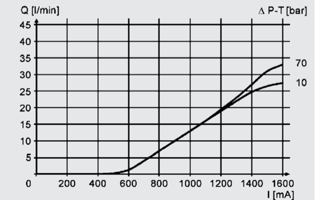
Q 26 spool
