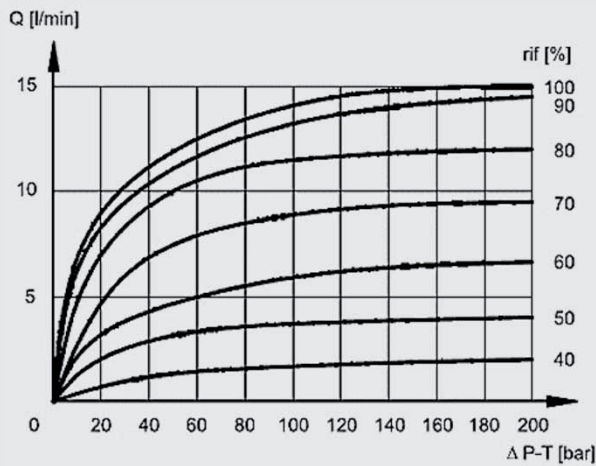
Q 08 spool
