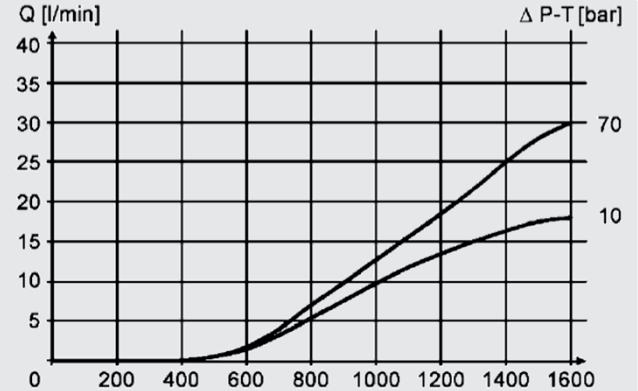
Q 16 spool
