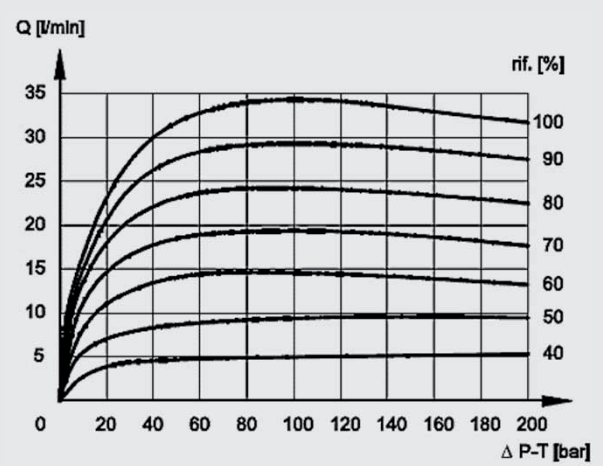
Q 26 spool
